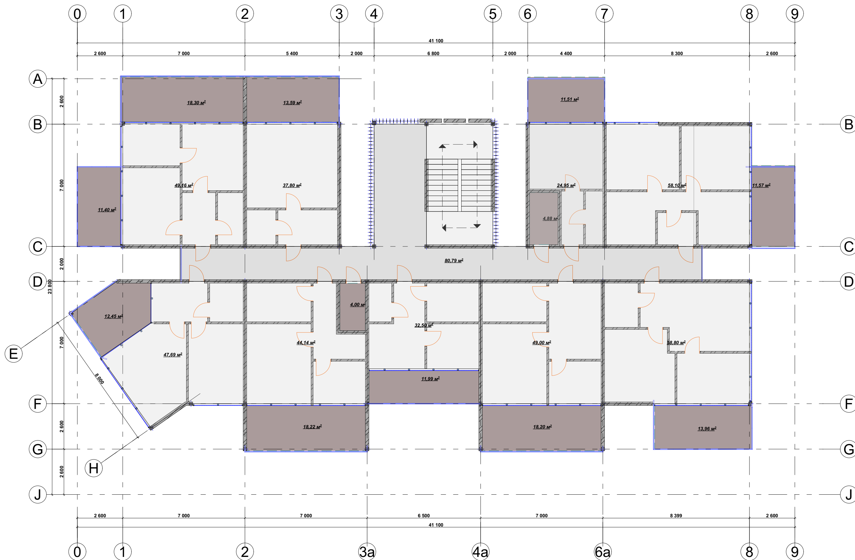
ПЛАН 3-ГО ПОВЕРХУ На відмітці +6.000
