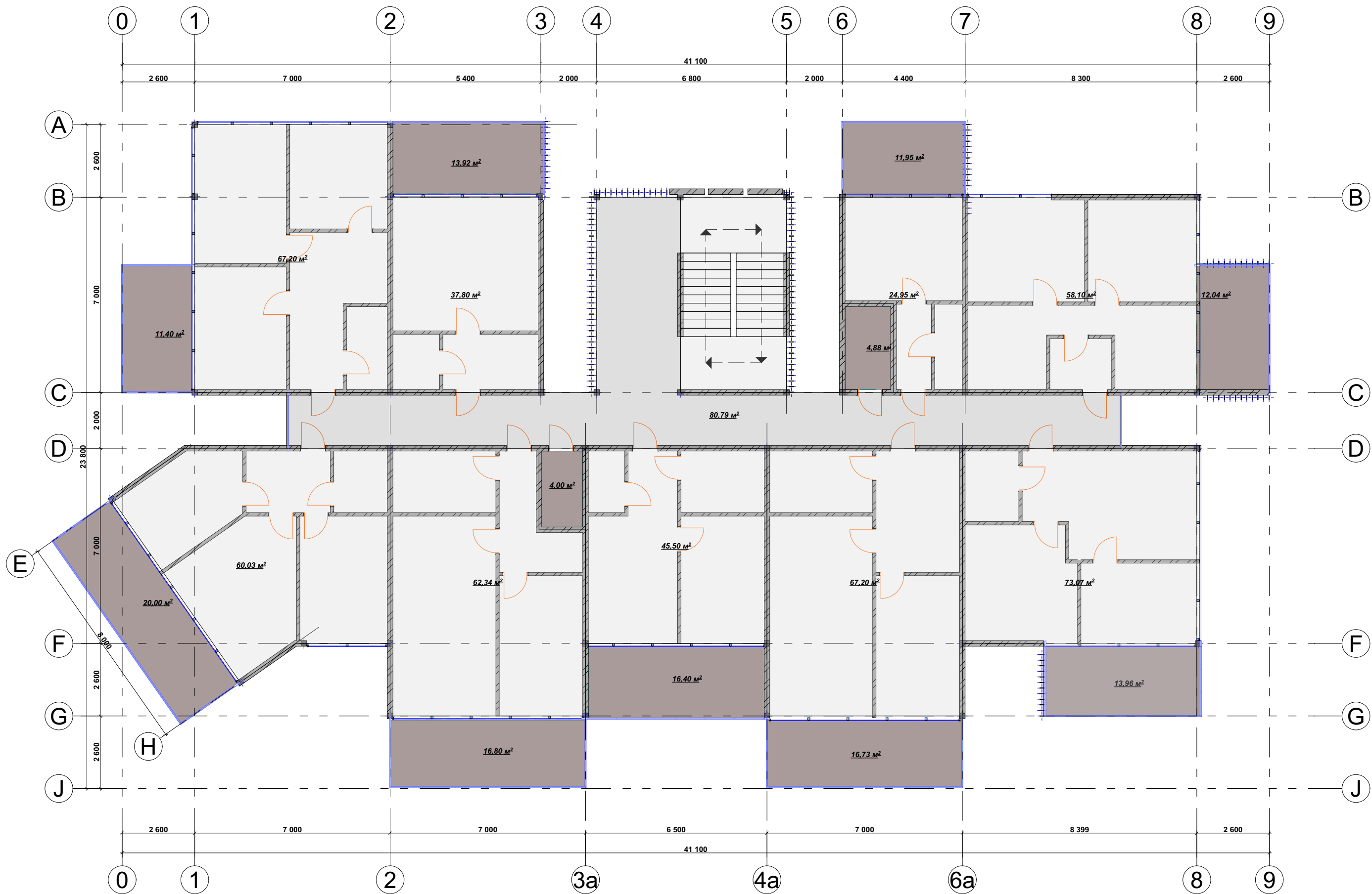
ПЛАН 2-ГО ПОВЕРХУ На відмітці +3.000
